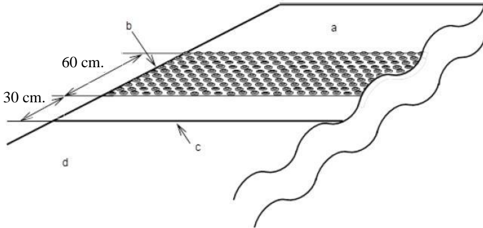
Şekil 6- Kaldırım rampası
