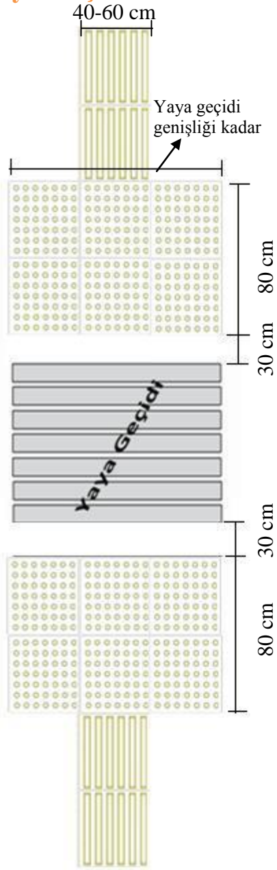
Şekil 9- Yaya geçidinde hissedilebilir uyarıcı yüzeý ölçüleri
