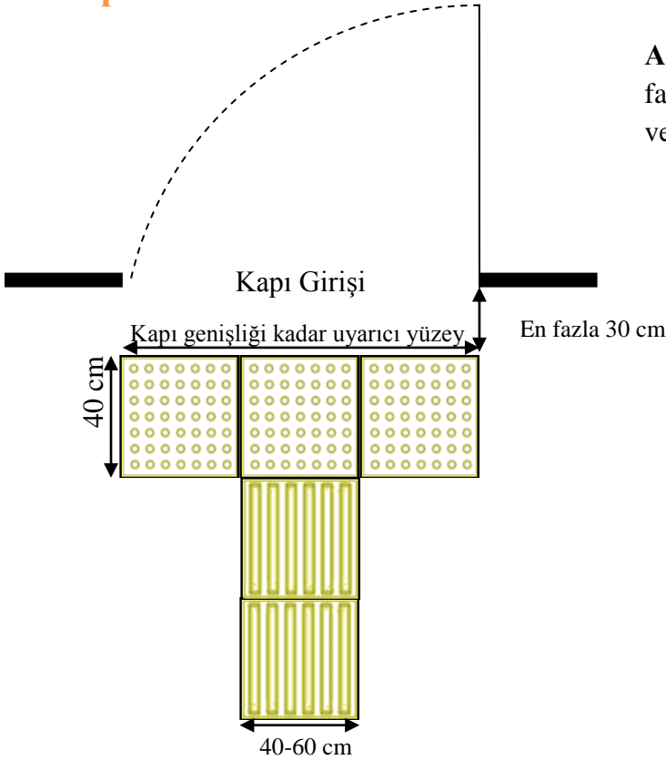
Şekil 13- Kapı öncesi hissedilebilir uyarıcı yüzey ölçüleri
